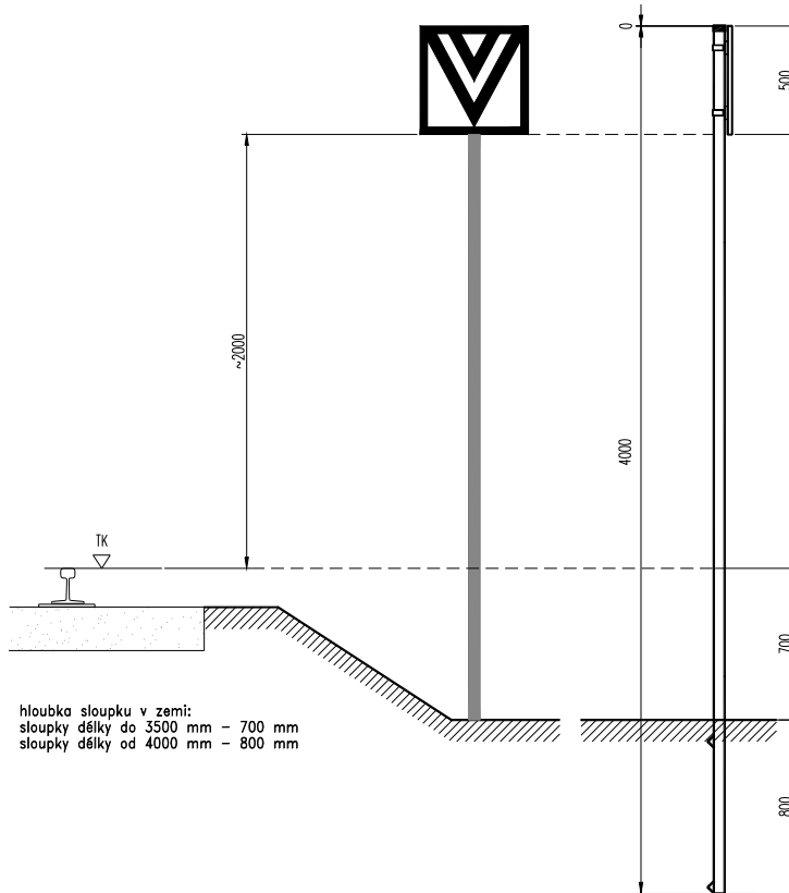
Sestava návěstidla s návěstí „Hranice pro návrat vozidel z širé trati”
