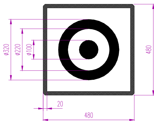
Návěst 39c
