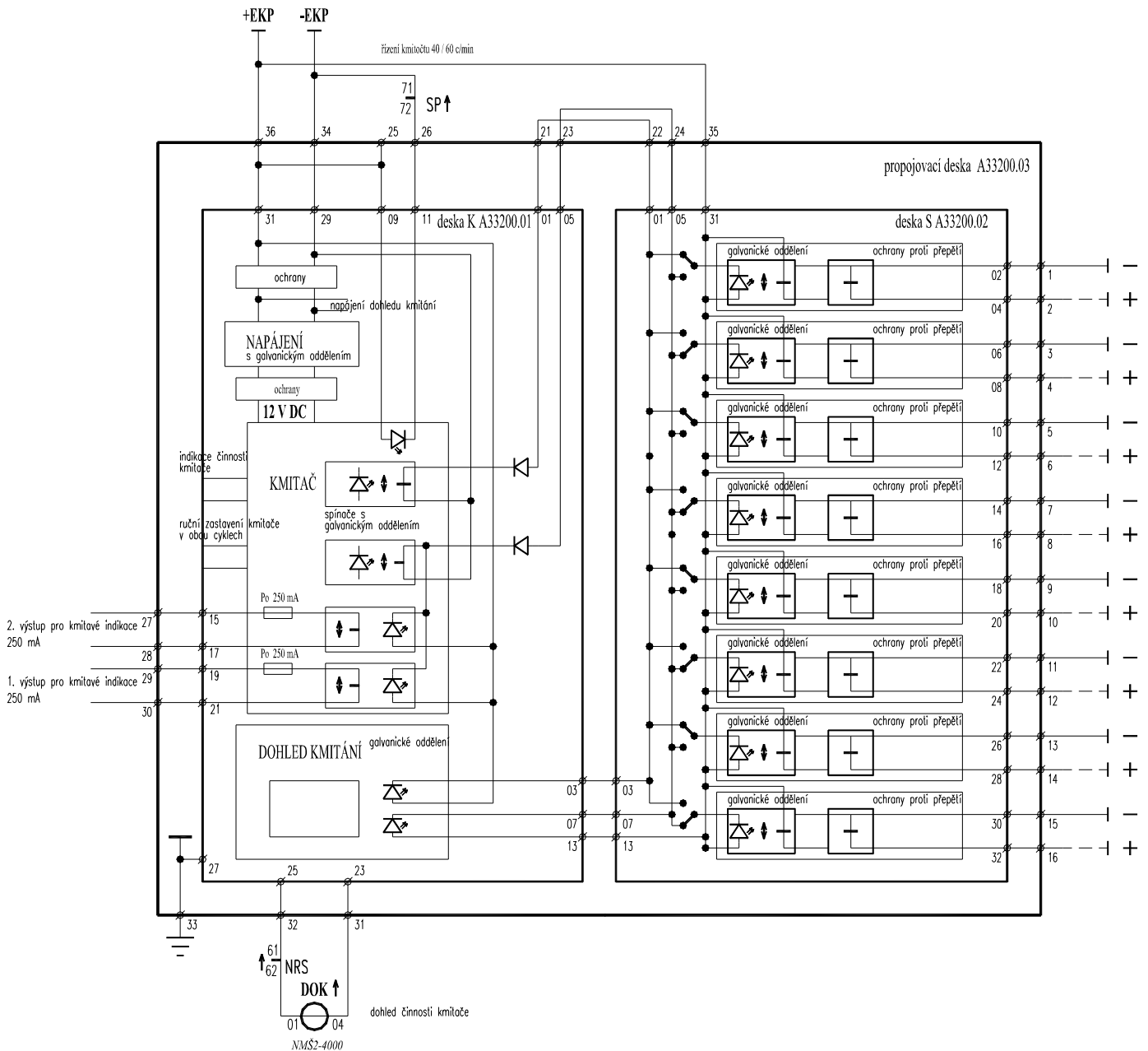
Blokové schéma EKPI č.v. A33200.c
